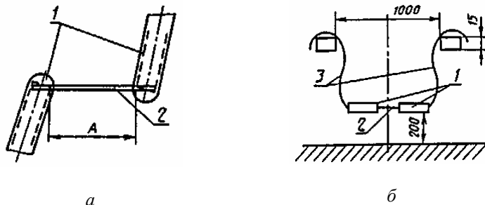
1 — электрододержатель; 2 — стержень; 3 — сварочный кабель Черт. 2
