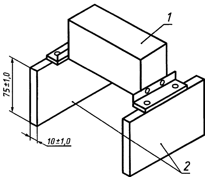
1 — трансформатор; 2 — деревянные подставки
