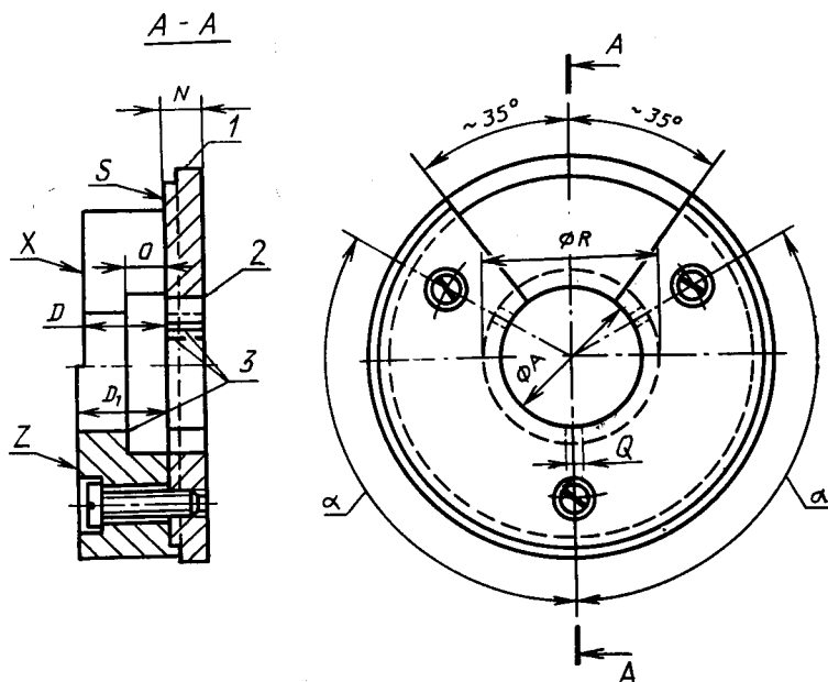
Проходной калибр для проверки цоколей типа ВА21 — 3(120°) на готовых лампах
