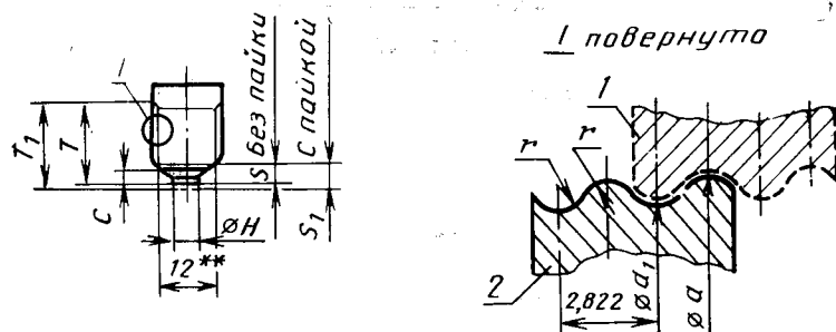
1 — патрон; 2 — цоколь
