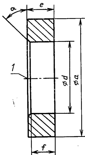
Непроходной калибр для проверки цоколей типов E10 и E40 на готовых лампах
