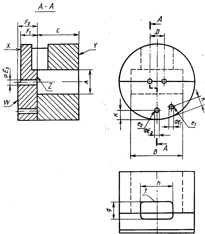
Калибр для проверки цоколя типа G5,3 на готовой лампе
