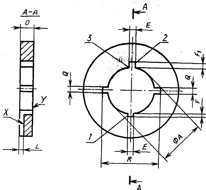
Калибр для проверки крепления цоколей типов B15d и B22d в патроне
