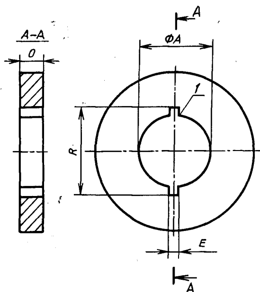
Калибр для проверки установки цоколей типов B15d и B22d в патроне
