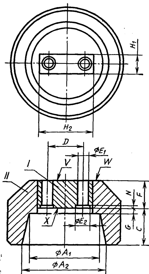
Проходной калибр для проверки цоколей типа G38 на готовых лампах
