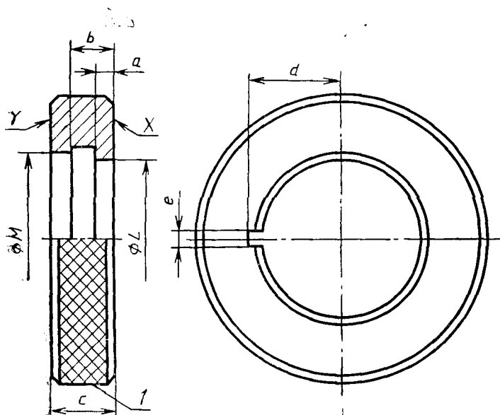
Проходной калибр для проверки фланца цоколя типа P45t — 4t на готовой лампе
