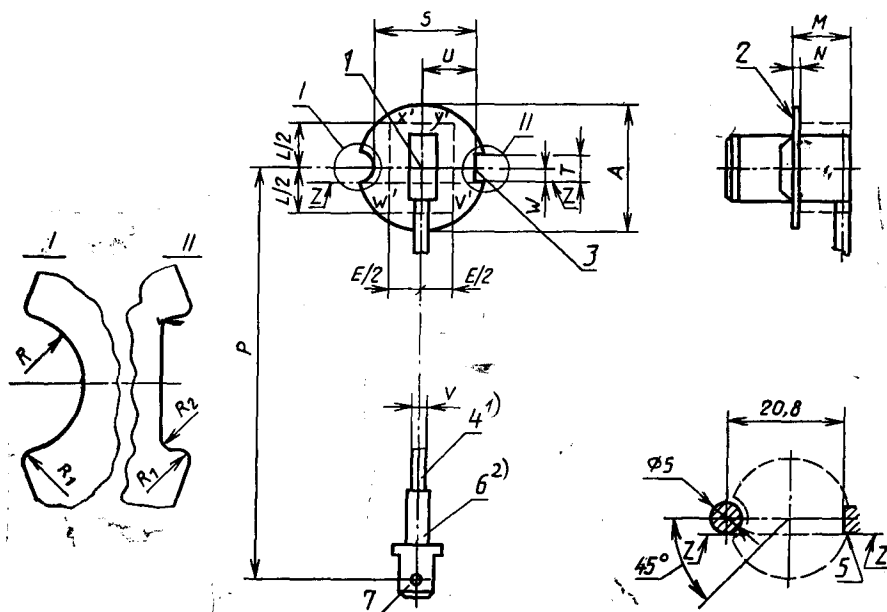
1 — центр фланца; 2 — базовая поверхность; 3 — исходный паз; 4 — изоляционный кабель (см. сноску 1); 5 — базовый ориентир; 6 — изоляционная часть (см. сноску 2); 7 — контактный штекер
