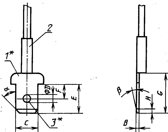
Контактный штекер цоколя типа PK22s
