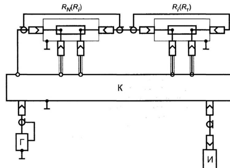
Рисунок Б.5 — Определение действительного значения сопротивления поверяемой УОМЭС с помощью двойного моста-компаратора УДМК-1М с автотрансформаторными плечами отношения
