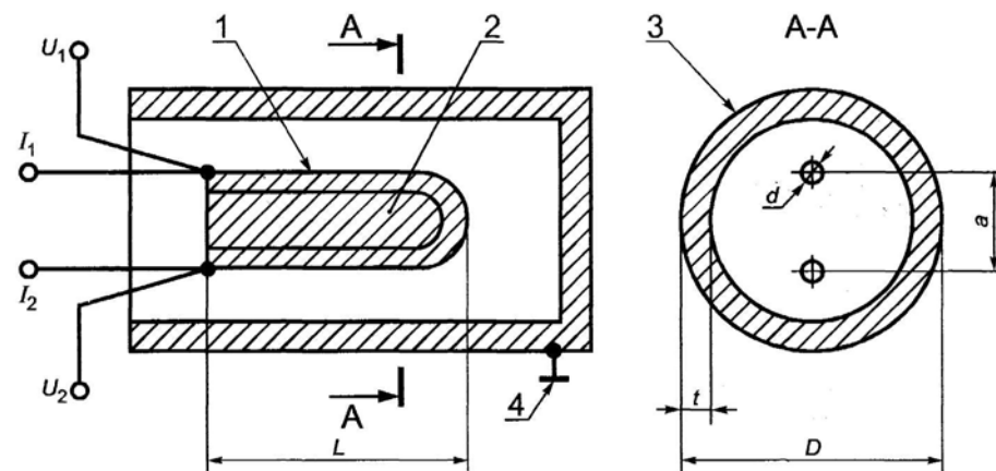
1 — резистивный элемент; 2 — диэлектрик; 3 — электростатический экран; 4 — зажим экрана; I_1, I_2 — токовые зажимы; U_1, U_2 — потенциальные зажимы
