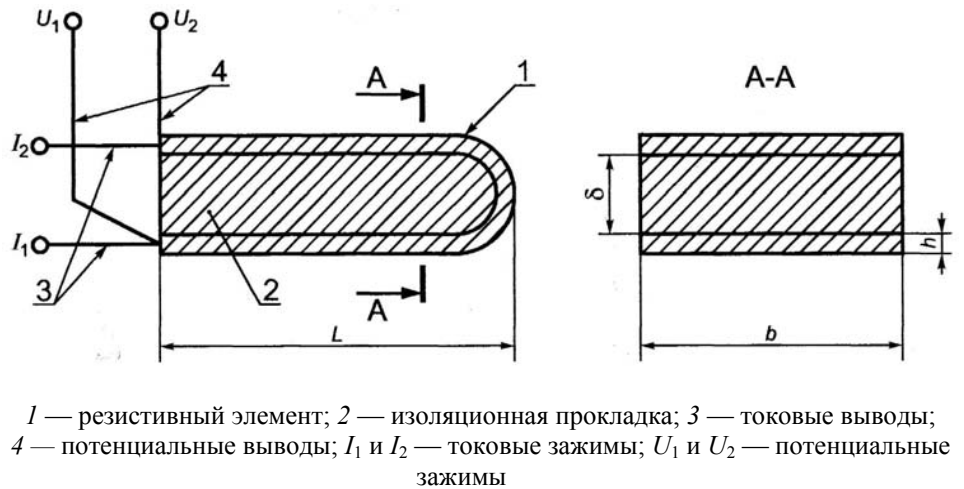
Рисунок Г.1 — Устройство низкоомного замещающего элемента
